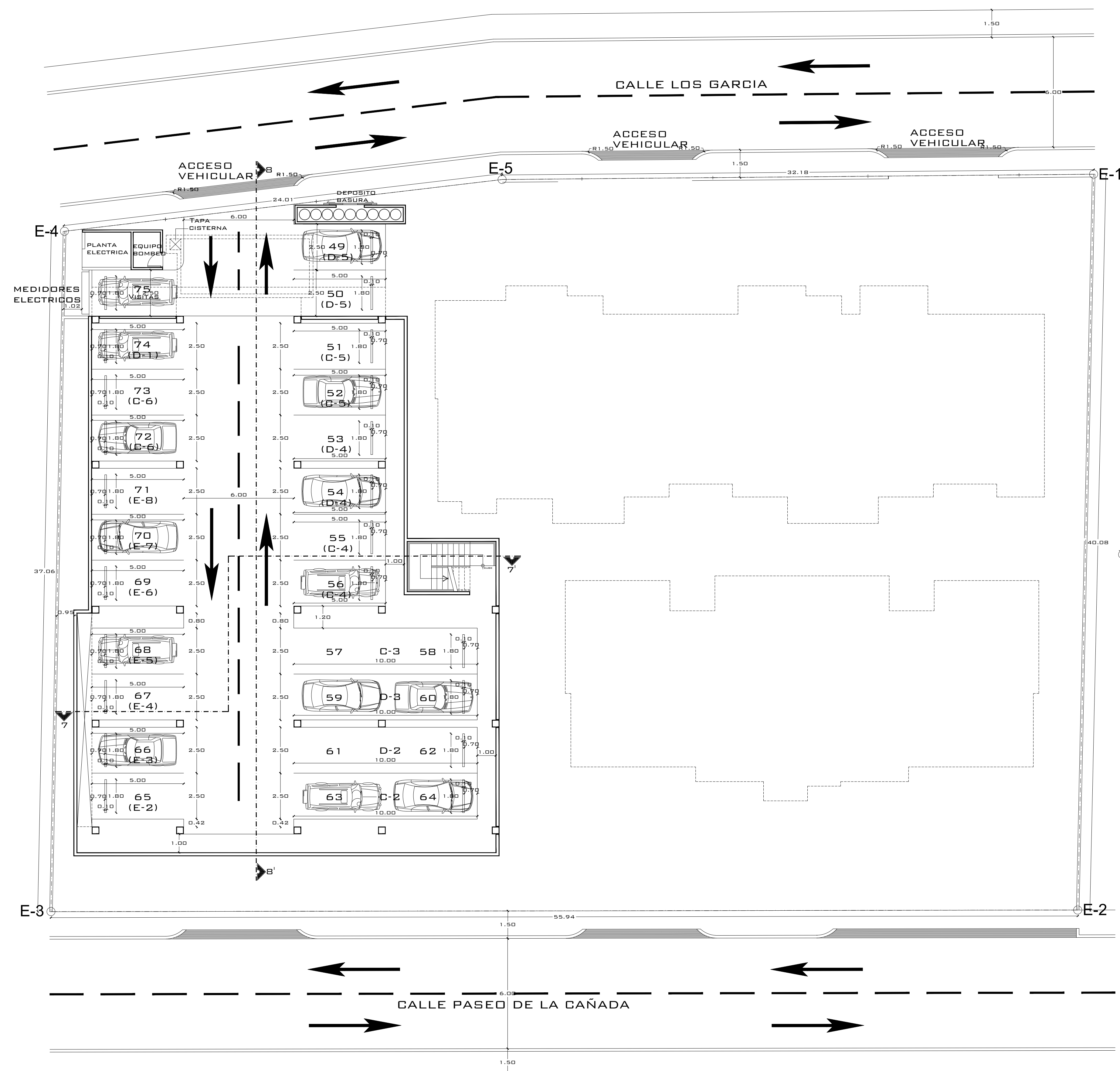
PLANTA AMUEBLADA DE PARQUEOS ESC. 1:125
